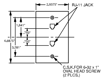
TPTE2
